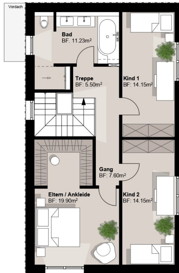
Haus Nr. 13 Grundriss OG, (5.5 Zimmer EFH) Brutto-Geschossfläche = 91.25m² 1:100
