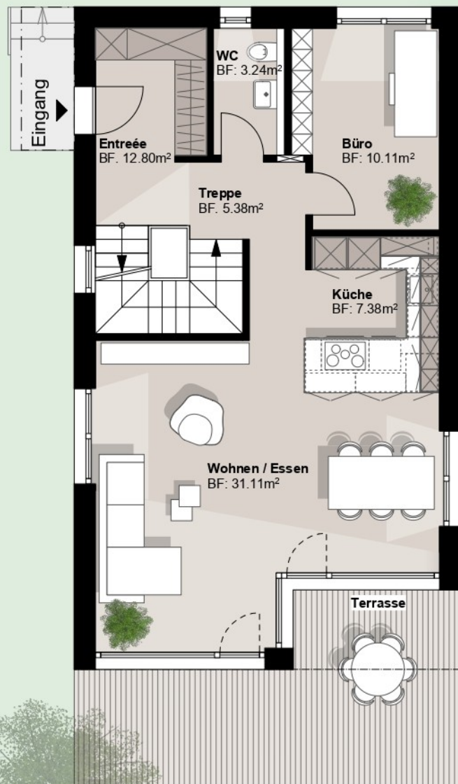
Haus Nr. 15 Grundriss EG (5.5 Zimmer EFH) Brutto-Geschossfläche = 86.50m² + Terrasse 20.81m² 1:100
