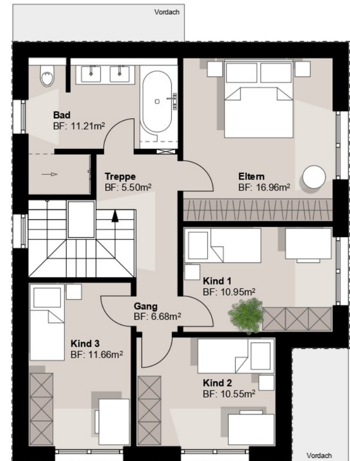
Haus Nr. 01, 02 Grundriss OG, (6.5 Zimmer EFH) Brutto-Geschossfläche = 92.30m 2 1:100
