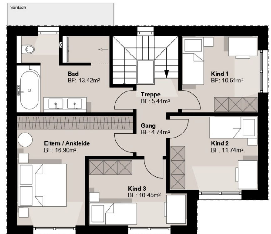
Haus Nr. 03, 08 Grundriss OG, (6,5 Zimmer EFH) Brutto-Geschossfläche = 92.30m 2 1:100
