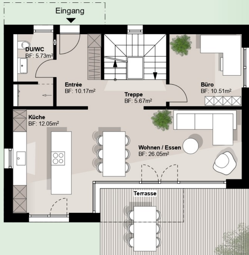
Haus Nr. 03, 08 Grundriss EG (6,5 Zimmer EFH) Brutto-Geschossfläche = 86.72m 2 + Terrasse 20.16m 2 1:100
