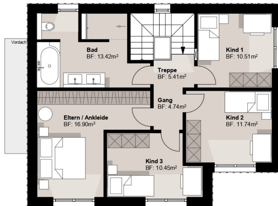
Haus Nr. 04 Grundriss OG, (6.5 Zimmer EFH) Brutto-Geschossfläche = 92.30m 2 1:100
