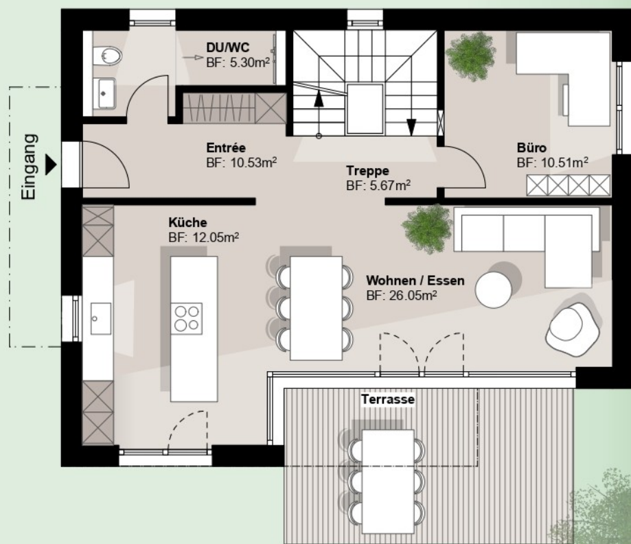
Haus Nr. 04 Grundriss EG (6.5 Zimmer EFH) Brutto-Geschossfläche = 86.72m 2 + Terrasse 16.71m 2 1:100
