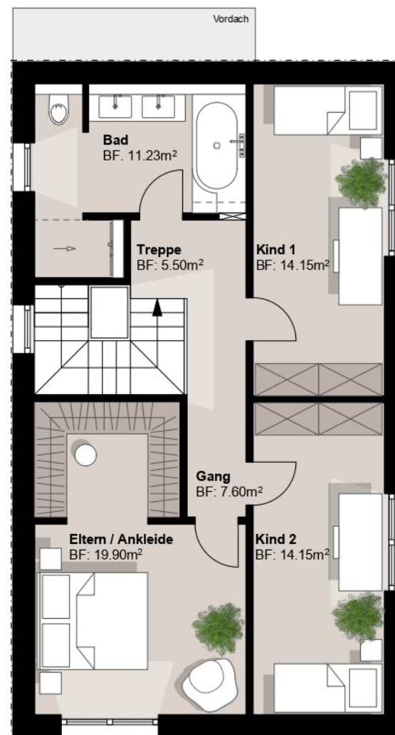
Grundriss Obergeschoss
